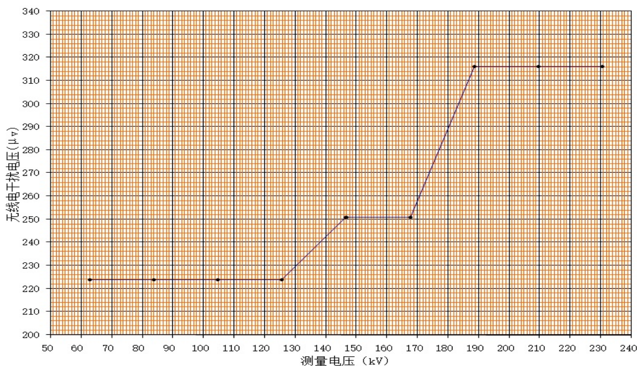
无线电干扰测量曲线
